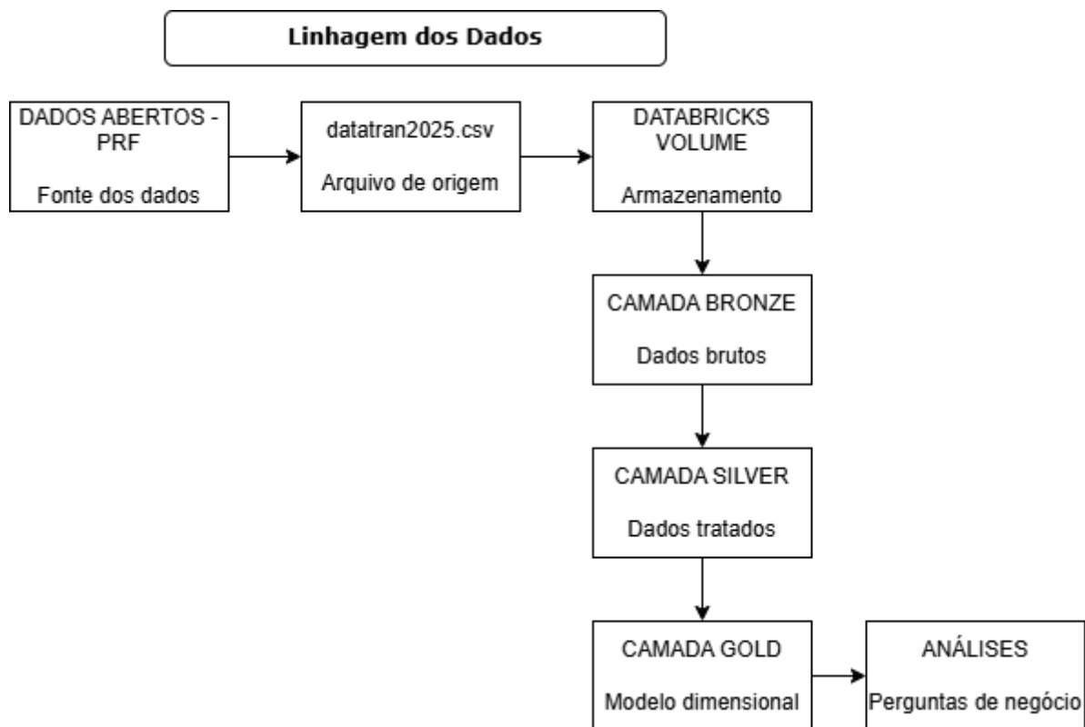
Figura 8 – Linhagem dos dados do pipeline.
